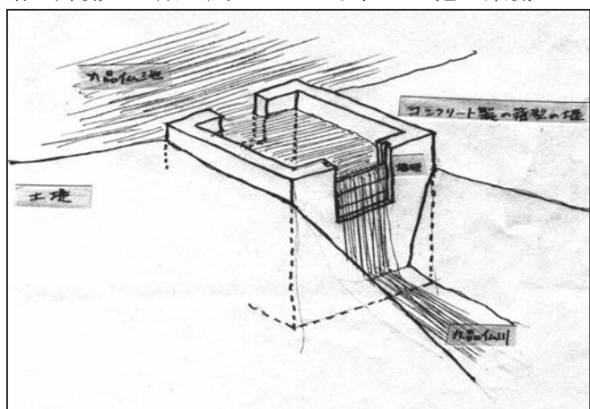
図2 水門の詳細
